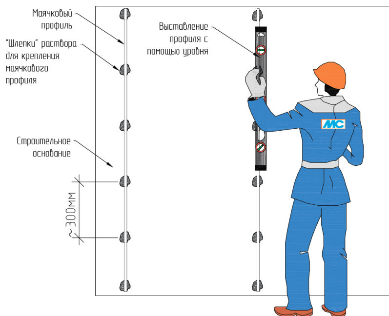
Рис.18. Монтаж маяка с помощью правила с уровнем
