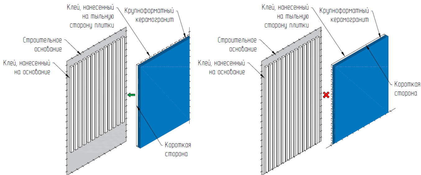
Рис. 28. Клей следует наносить в одном направлении на основание и на плитку
