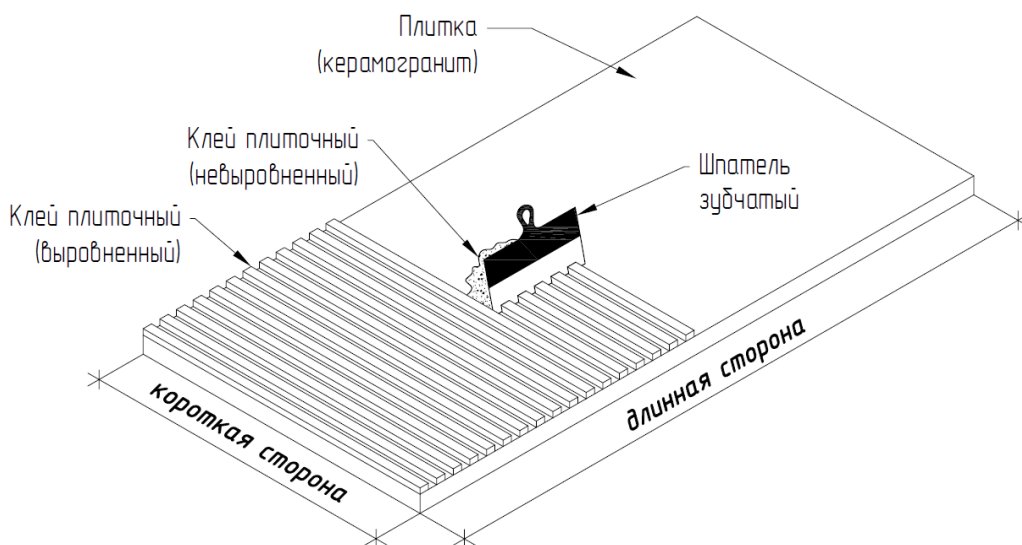
Рис. 27. Нанесение плиточного клея на плитку
