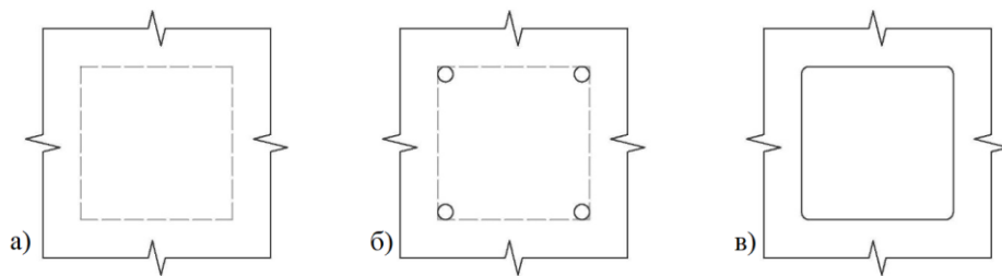
Рис. 30. Резка прямоугольных отверстий
