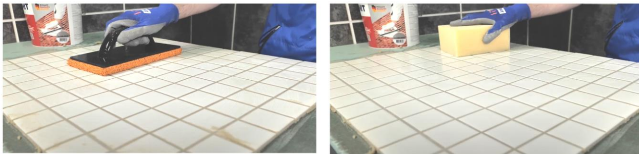
Рис. 38. Диагональными движениями шпателя убрать с поверхности плитки излишки затирки
