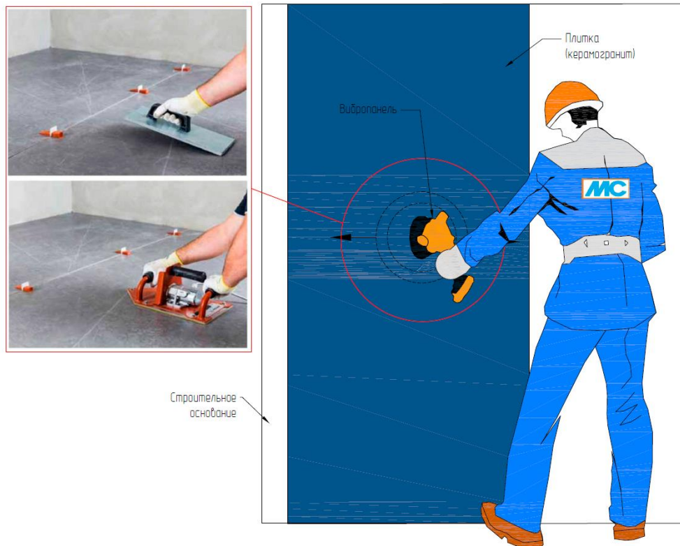
Рис. 32. Увеличение адгезии плитки с основанием вибрированием или простукиванием
