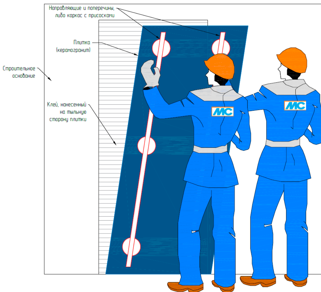
Рис. 31. Монтаж крупноформатного керамогранита
